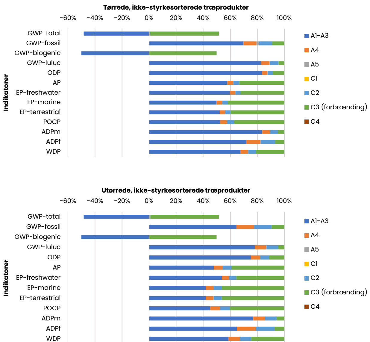
Figur 1 Bidragsanalyser for tørrede (øverst) samt utørrede (nederst) ikke-styrkesorterede træprodukter. Graferne er vist med forbrændings scenariet for C3.
