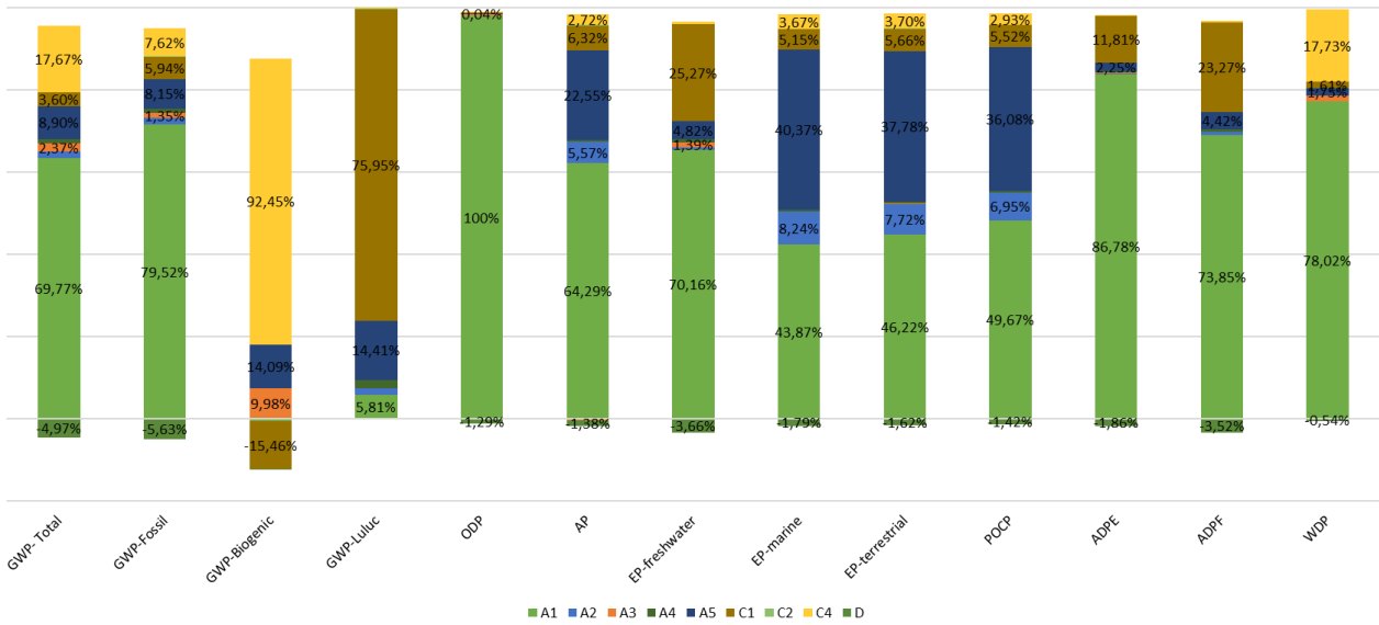
Dominansanalyse SAERTEX-LINER® H2O Ø 300 mm / 4,3 mm
