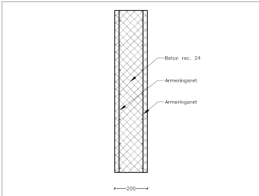
Tværsnit af 200 mm betonelement fra SHT A/S
